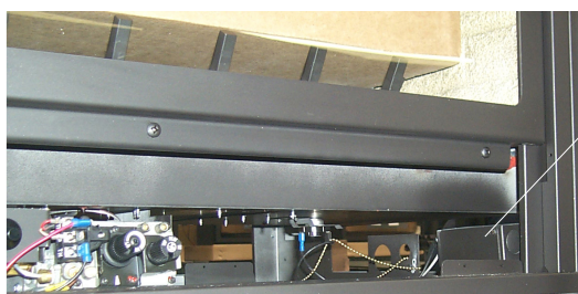
Retirer le couvercle pour accéder au bloc de jonction
