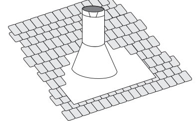
Schéma 4 : Installer la portion supérieure du solin au-dessous des matériaux de toiture et ne pas la fixer avant l'installation du conduit de cheminée. De petits ajustements pourront ainsi être effectués par la suite.
