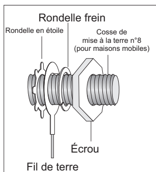
Illustration détaillée de la mise à la terre
