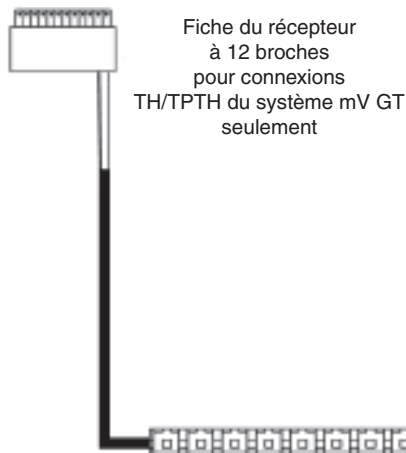
Récepteur mural
