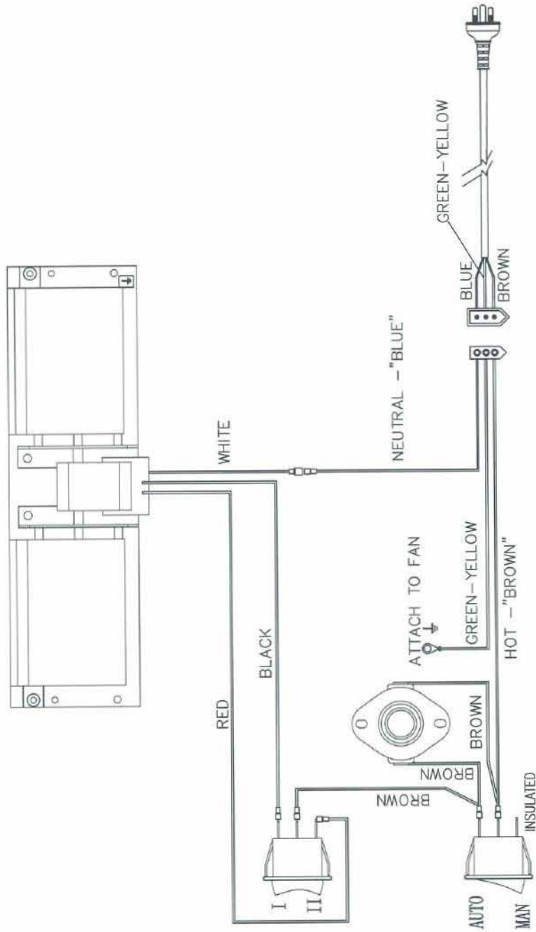
Internal Fan Wiring Diagram (240V)
