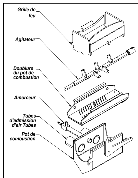
Figure 8 : Dispositif du pot de combustion pour le GCI60-2
