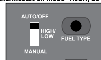
Figure 5 : Interrupteur thermostat en mode "AUTO/OFF"
