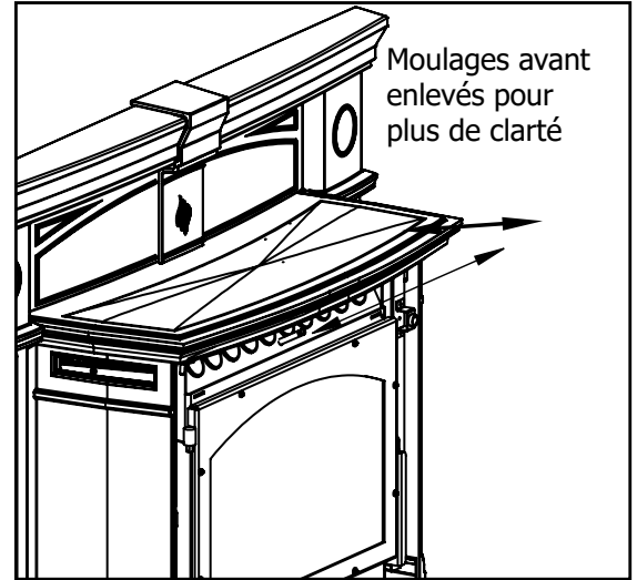
Figure 9 : Nettoyage de l'échangeur thermique du GCI60
