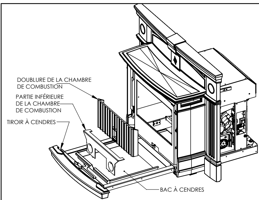
Figure 10 : Passages de l'évacuation du modèle GCi60
