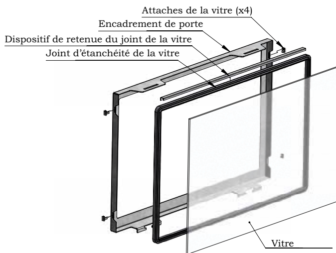
Éléments de la porte
