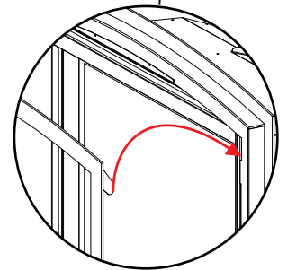
Installer le cadre extérieur Vignette par-dessus le cadre intérieur Vignette
