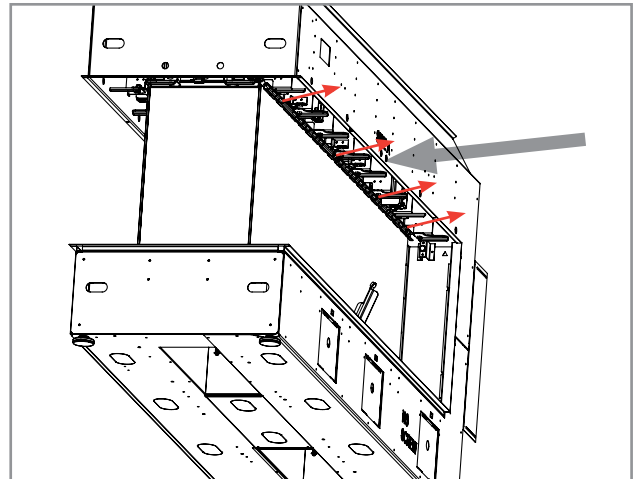
Lorsque les attaches supérieures sont en position ouverte, utiliser vos mains pour tirer les deux rails du joint d'étanchéité de la vitre vers vous.
