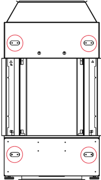
Trous d'accès pour retirer les supports de transport
