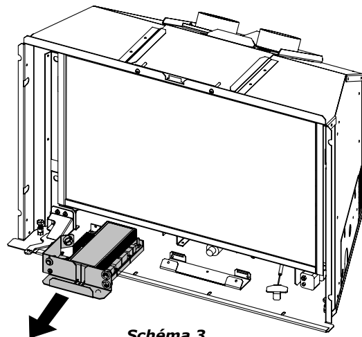
Schéma 3
