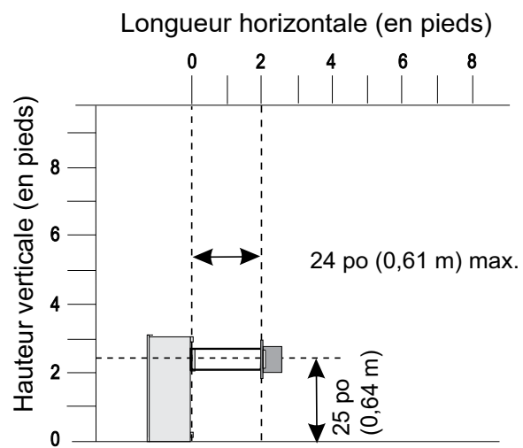
Évacuation à l'arrière
