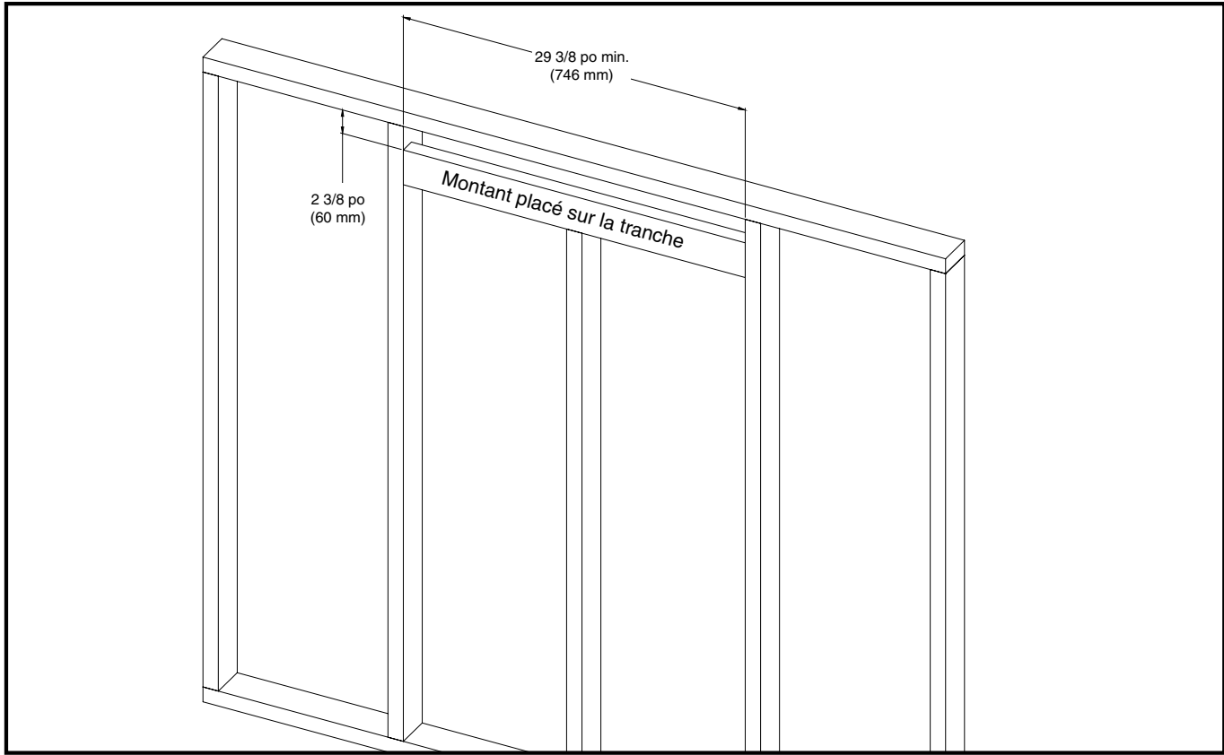
VUE LATÉRALE
