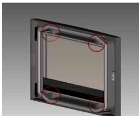
Emplacement des vis des attaches de la vitre
