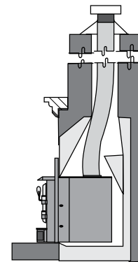
Hauteur de cheminée recommandée depuis la partie supérieure de la buse de cheminée : 15 pieds min. (4,6 mètres)
