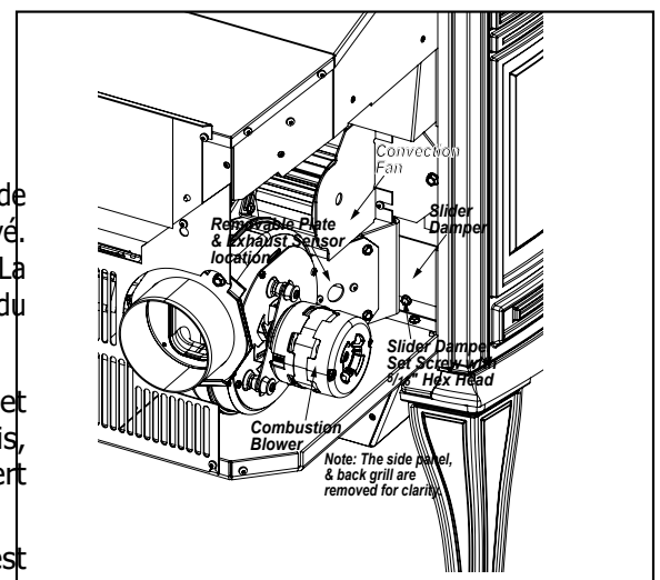
Figure 6: Plaque de l'amortisseur à glissière dans l'unité.
