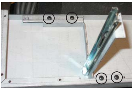
emplacement des vis HZ42ST
