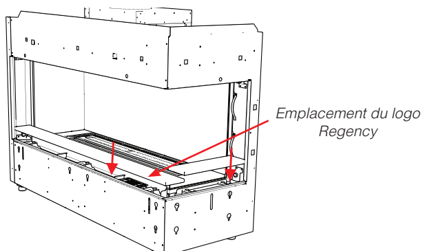
Installation des panneaux de la base externe
