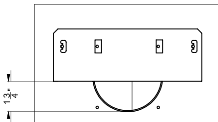
Position 2 (Réducteur d'air à 1,75 po)
