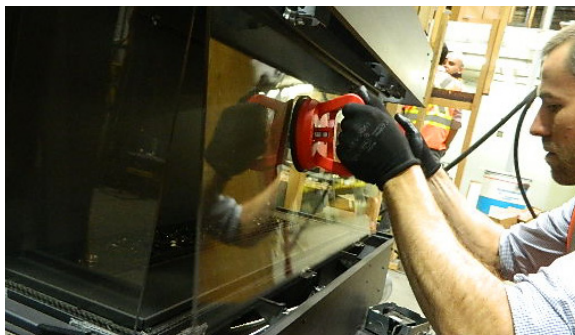
Manipuler le panneau avant à l'aide des ventouses fournies
