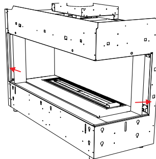
Installation du panneau externe latéral
