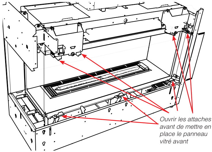
Illustration Modèle CC40LE
