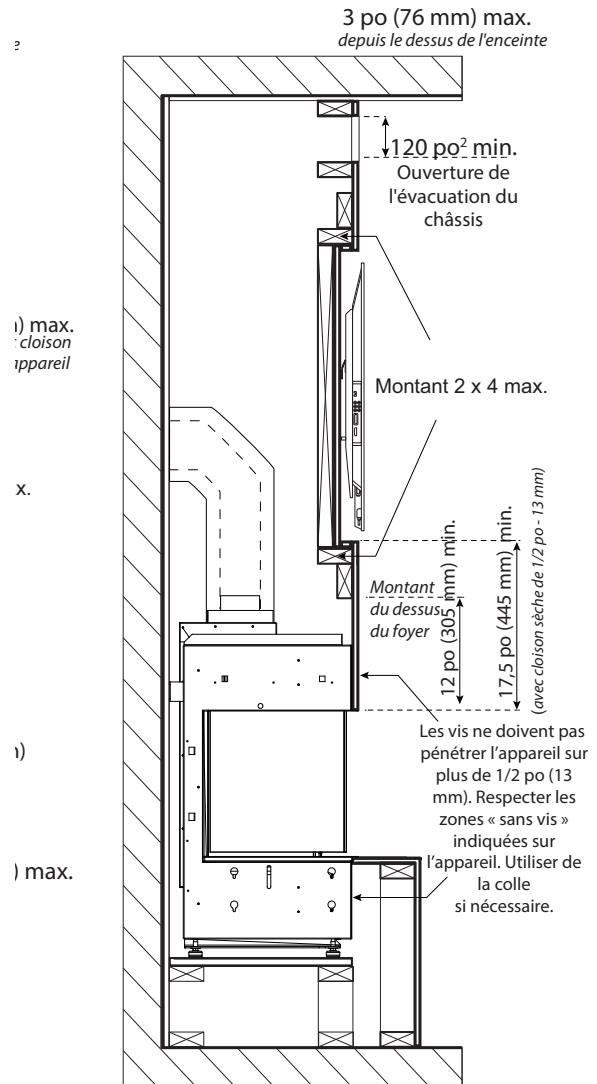
Encastrement TV affleurant au mur avec une cloison sèche de 1/2 po (13 mm)
