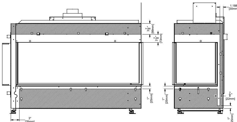
Modèle CC40RE - Vis uniquement dans la zone ombragée
