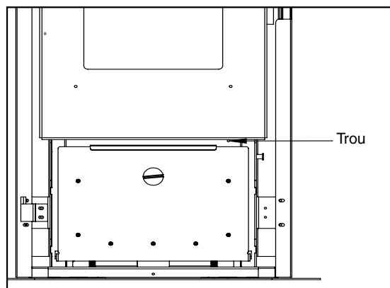
Trou d'essai du manomètre
