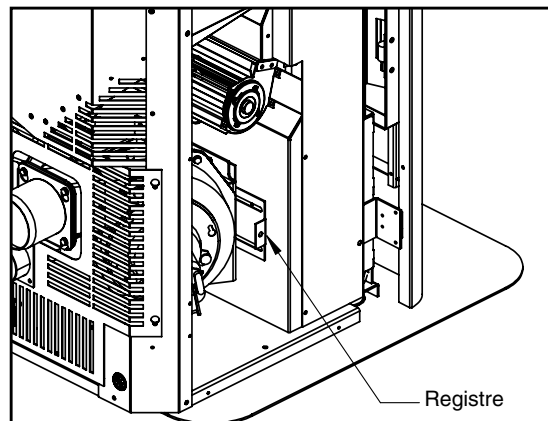
Réglage du registre à glissière
