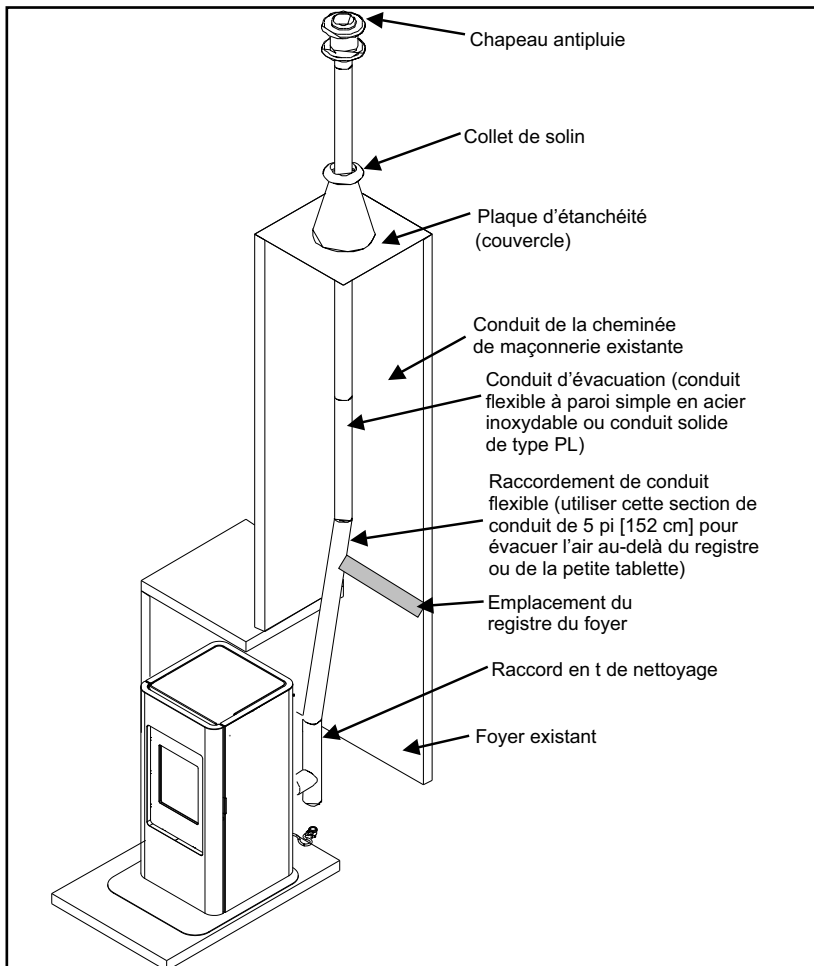
Aperçu de l'installation de l'âtre du poêle autoportant
