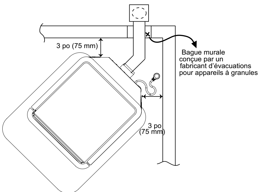
Installation en angle
