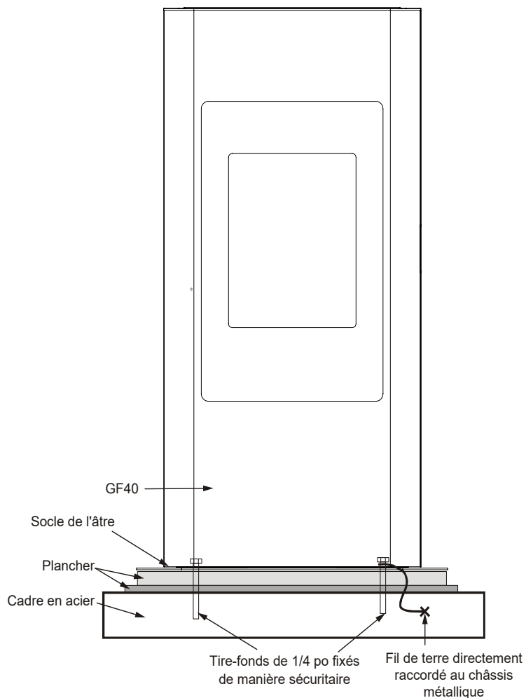
Installation dans une maison mobile
