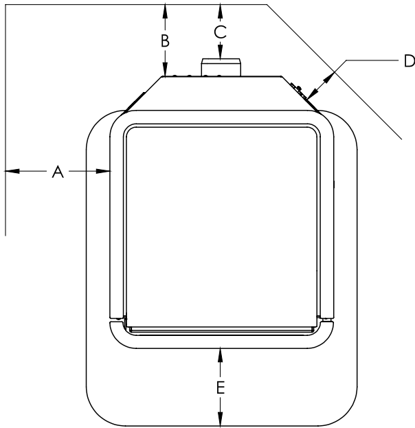
Dégagements de l'installation minimale
