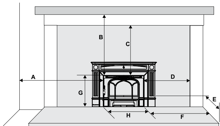
Schéma des dégagements requis pour les installations
