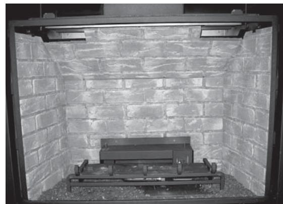
Panneau de brique installation complète
