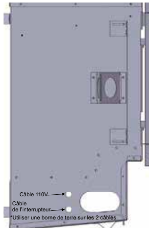
Modèle HZO42
