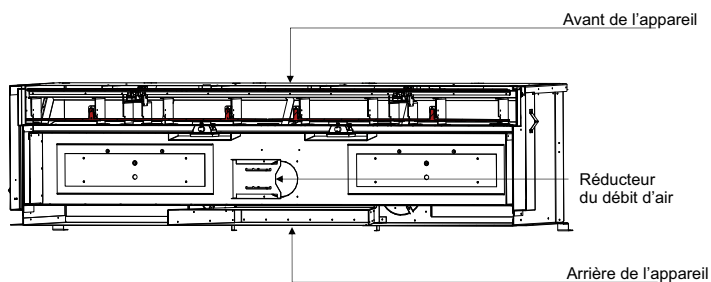
Section transversale illustrant le plafond de la chambre de combustion depuis l'intérieur
