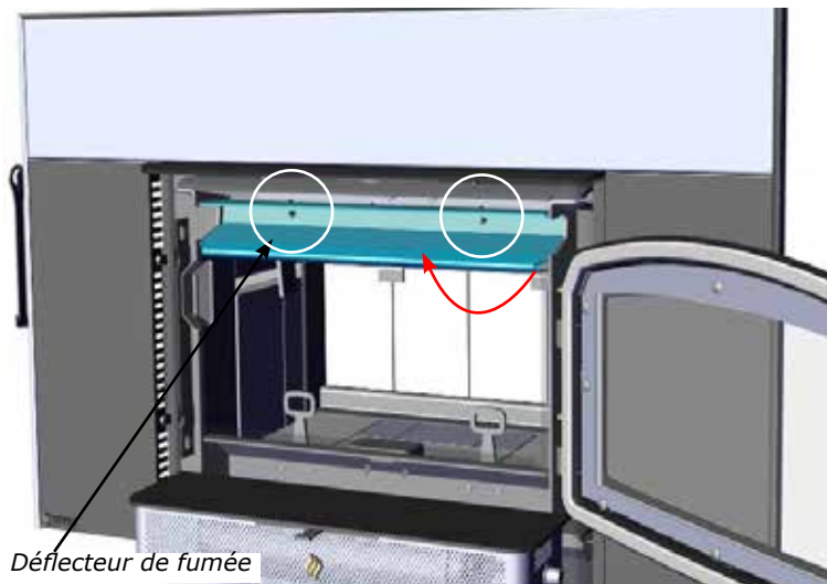
Le déflecteur de fumée est installé par l'ouverture de la porte dans l'emplacement indiqué sur le schéma.
