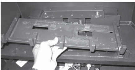
Dévisser les deux vis, glisser le brûleur vers la gauche et le soulever.
