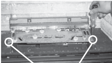
Dévisser les deux vis, glisser le brûleur vers la gauche et le soulever.
