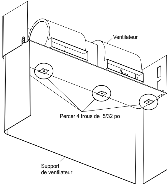
Schéma 9 : Vue arrière/du dessous
