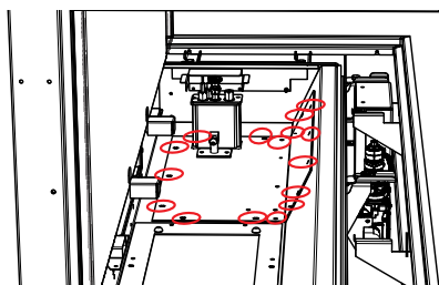
Retirer les 16 vis qui maintiennent le plateau de la valve
