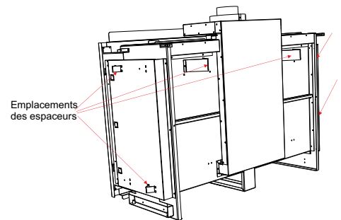
Modèles CC40LE/CC40RE
