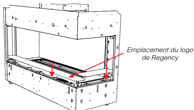
Installation des panneaux externes de la base
