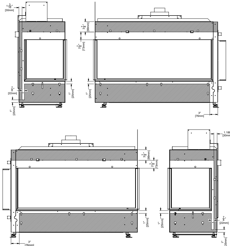
Modèle CC40LE - Vis uniquement dans la zone ombragée
