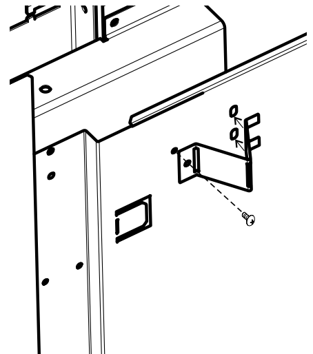
Modèles CC40LE/CC40RE
