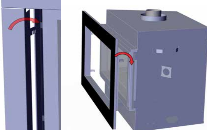
Schéma 1 - Installation du contour vitré
