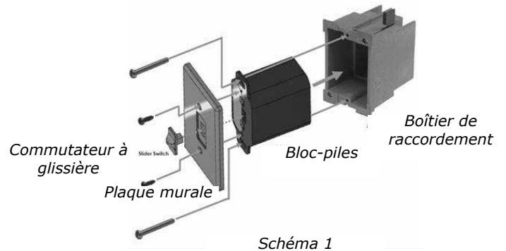
Boîtier de raccordement basse tension
