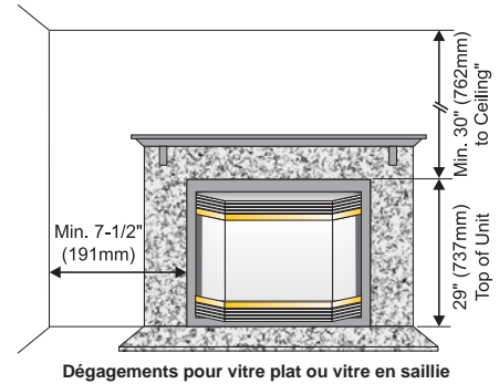
Dégagements pour vitre plat ou vitre en saillie
