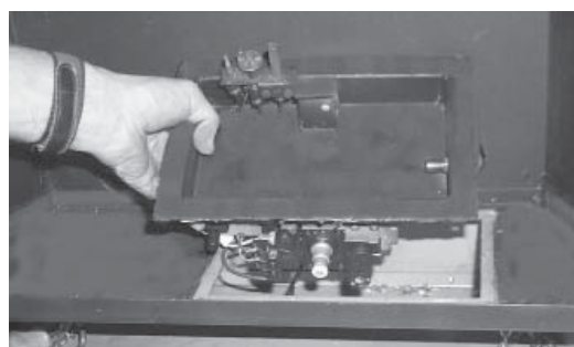
Schéma 3: soulever le plateau de la soupape
