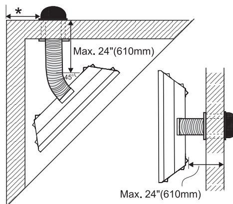
Dégagement d'évent minimum et maximum
