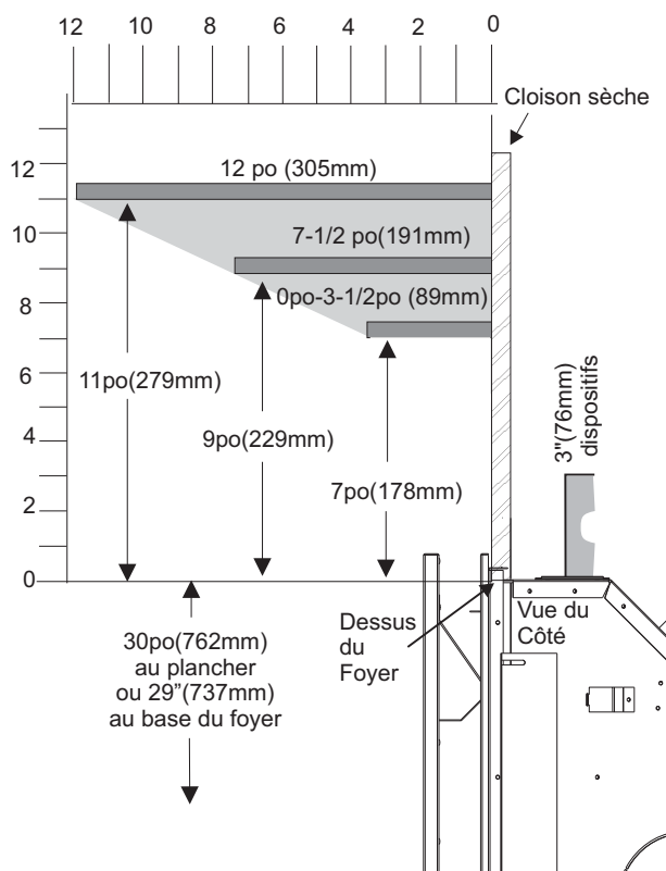
Dégagement de manteau avec la façade contemporaine
