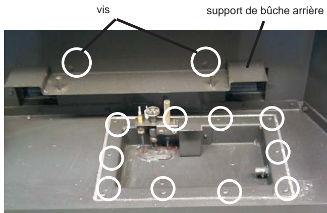
Le schéma 2: support de bûche arrière & plateau de la soupape
