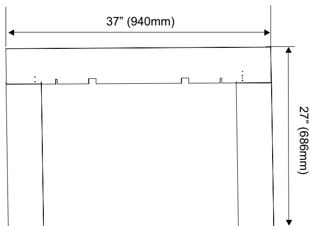
Modèle Ci1150-1 sur mesure - Dimensions minimales
