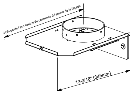
ADAPTEUR DE CHEMINÉE STANDARD (172-942) 6 po (152 mm) de diamètre
