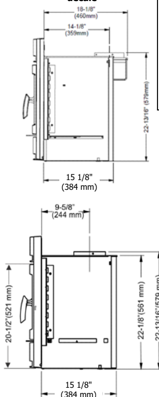
ADAPTEUR DE CHEMINÉE DÉCALÉE (172-946) 6 po (152 mm) de diamètre
