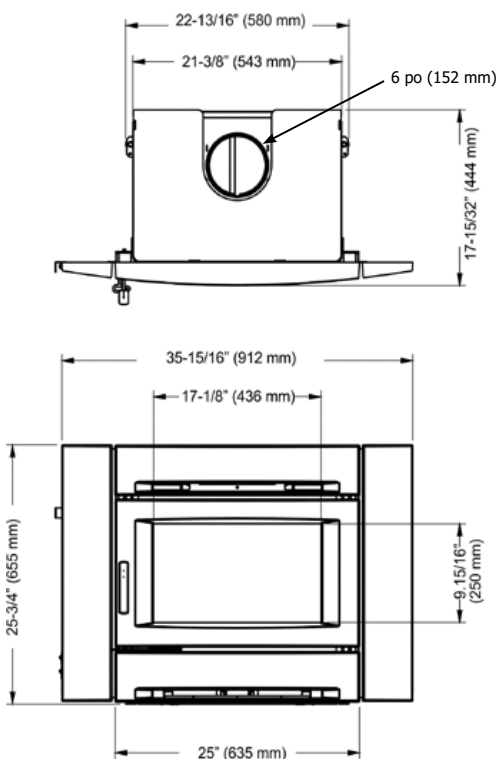
ADAPTEUR DE CHEMINÉE STANDARD (172-942) 6 po (152 mm) de diamètre
