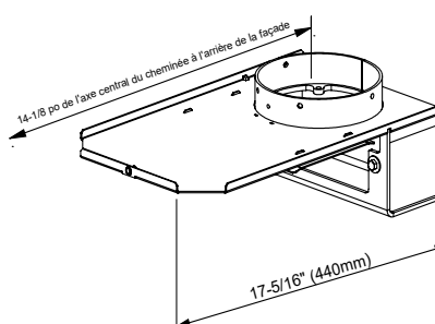
ADAPTEUR DE CHEMINÉE DÉCALÉE (172-946) 6 po (152 mm) de diamètre
